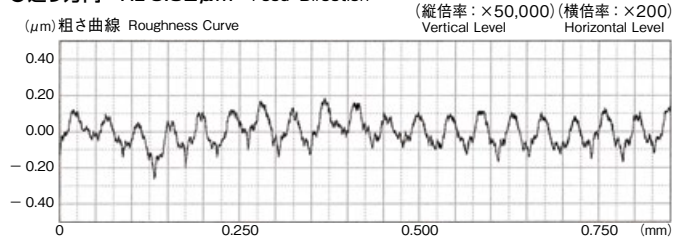
●ピック方向 R_z 0.21\mu\text{m} Pick Direction
