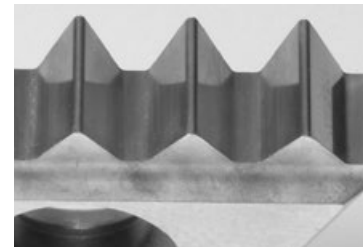
正常摩耗のインサート Normal wear of insert
