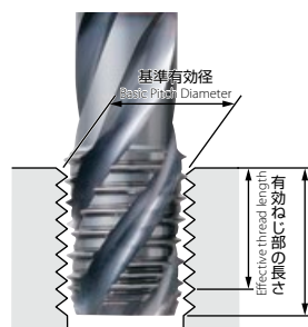
タップによる加工 Processing by tap
