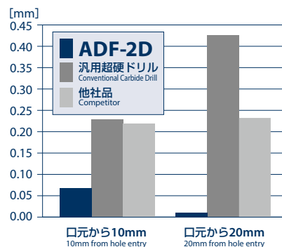
■倒れ量 (口元から1mmの値を基準として) Fallen amount (based on the value of 1 mm from hole entry)
